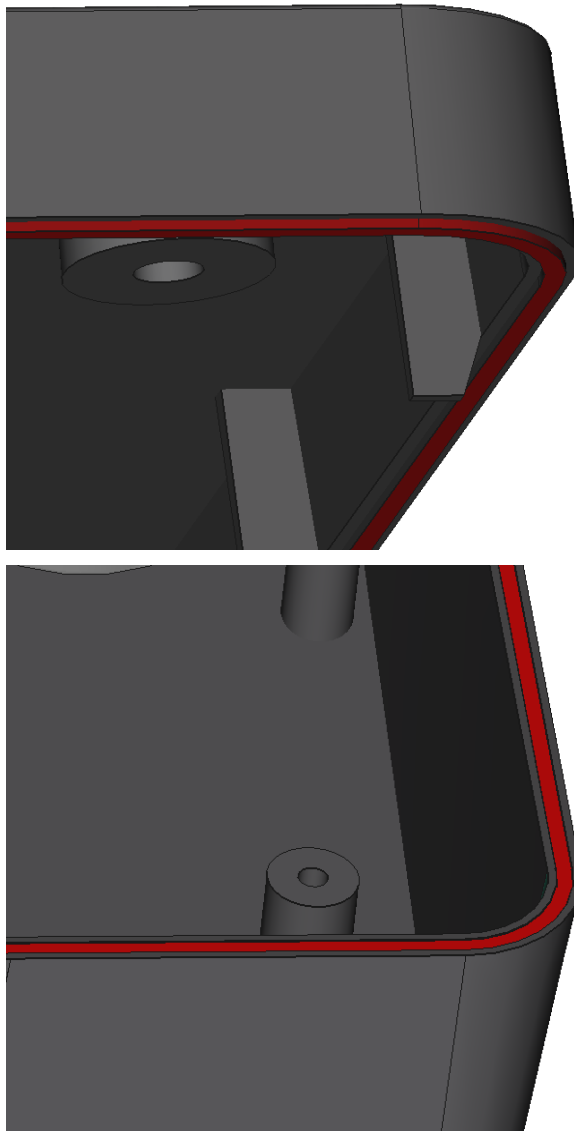
Рисунок 10 – Выемка с уплотнительной резинкой на корпусе считывателя и выступ на задней крышке.
